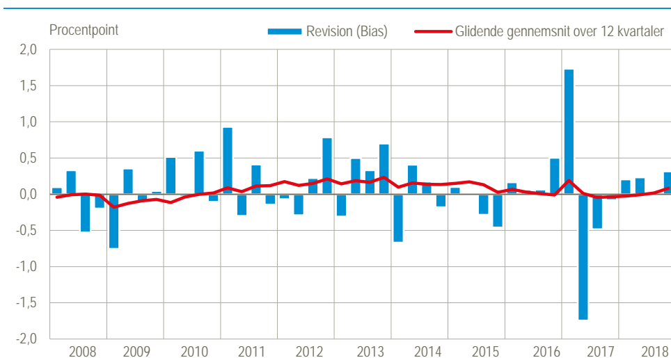
Figur 1. Revision (bias)
